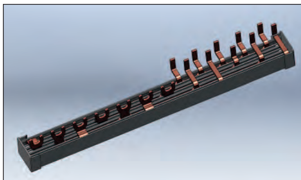
Einspeisung (FI) vierpolig, Abgang dreipolig, 5 Abgänge L + N
