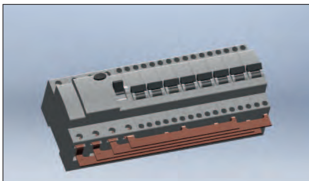
FI (Gabelanschluss) mit zweipoligen LS-Schaltern (ohne Isolierung)
