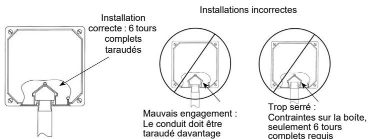
Figure 5 : Installation typique du panneau
