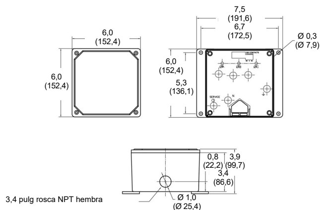
Figure 11 : Dimensiones generales
