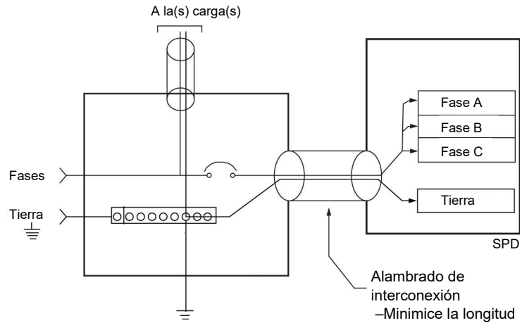
Figura 3: Alambrado del SPD para las configuraciones en delta
