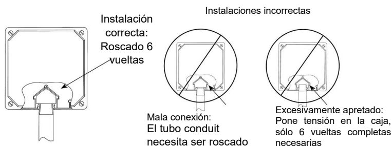
Figura 4: Instalación del tubo conduit
