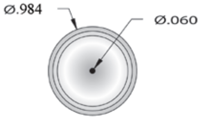
1/8" MINI T.C.
