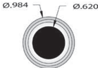
3/4" MINI T.C.
