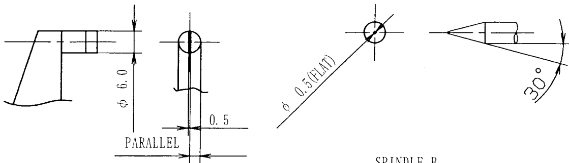
SPINDLE B
