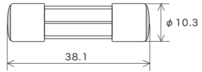
Scale: 1/1 (mm)
