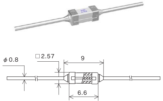
Scale: 2/1 (mm)
