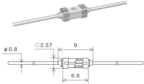
Scale: 2/1 (mm)
